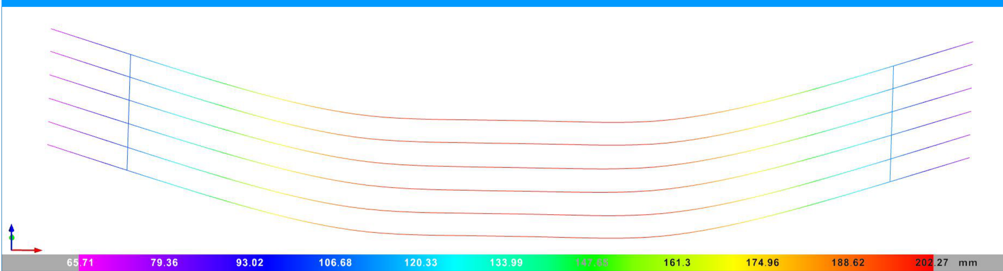
VENTANA DE ISOVALORES Y DEFORMACIONES EN VARALES
