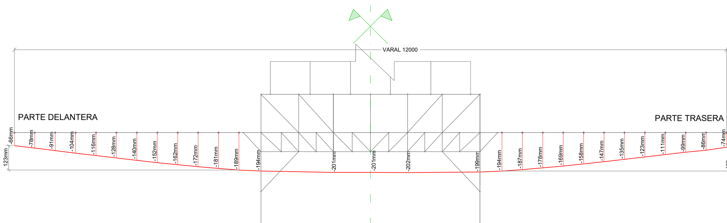
DEFORMACIÓN TEÓRICA DEL VARAL PARA TALLAJE DE PORTADORAS Y PORTADORAS
