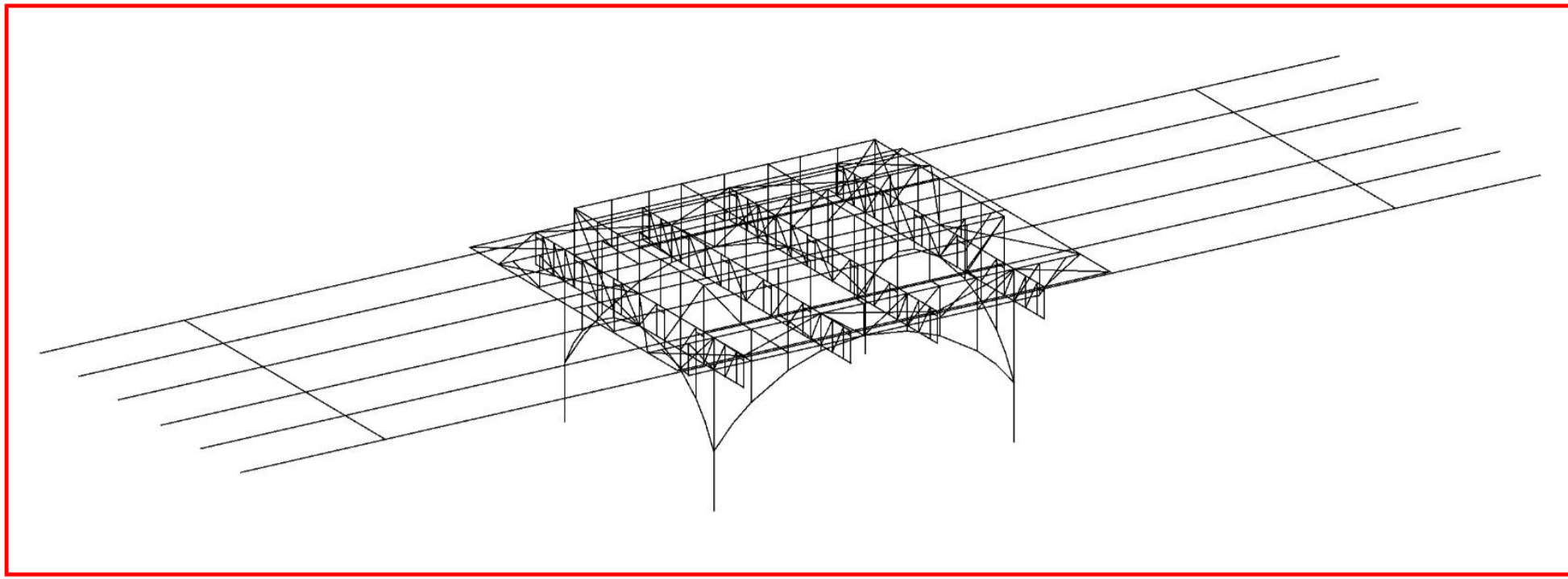
MODELO 3D ESTRUCTURA COMPLETA DEL TRONO EN SOFTWARE DE CAD
