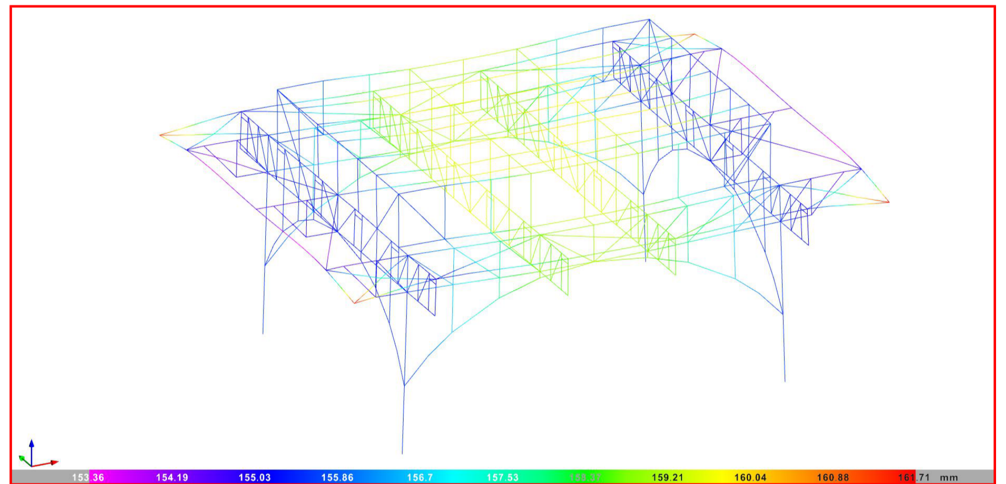
DIAGRAMA DE ISOVALORES: DEFORMADA DE LA ESTRUCTURA DE LA MESA. TRONO EN MOVIMIENTO
