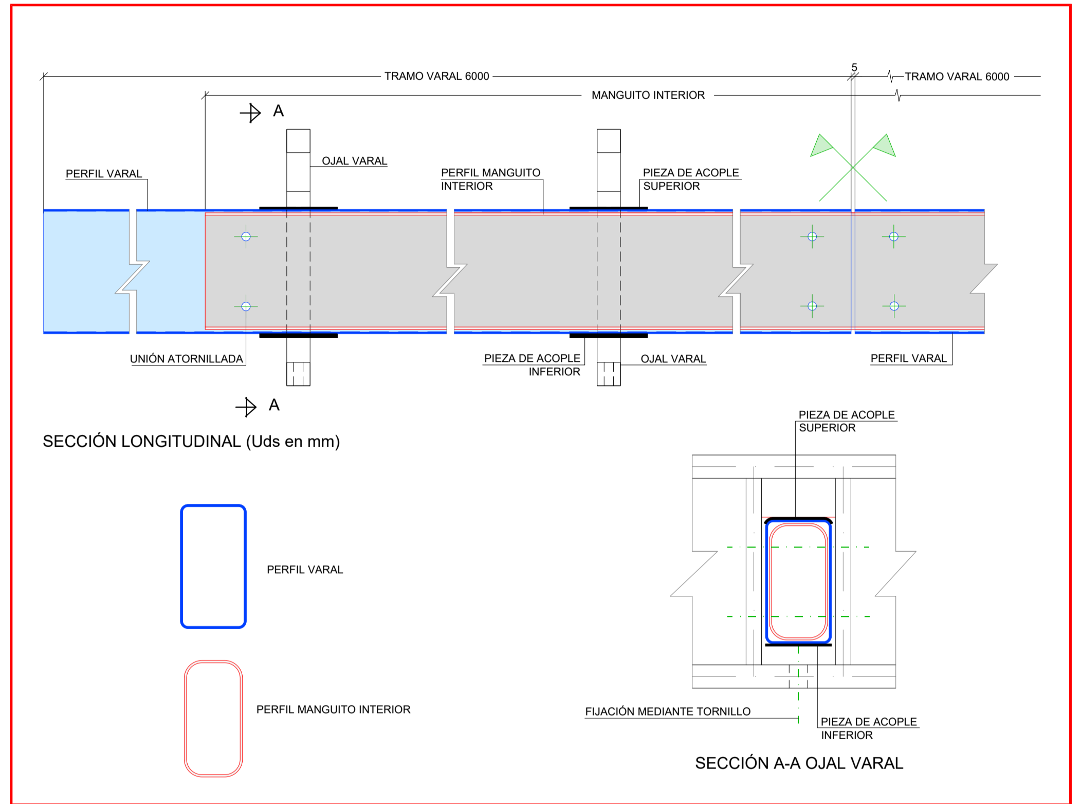
DETALLE MONTAJE DE VARALES MEDIANTE CONEXIÓN CON MANGUITO INTERIOR
