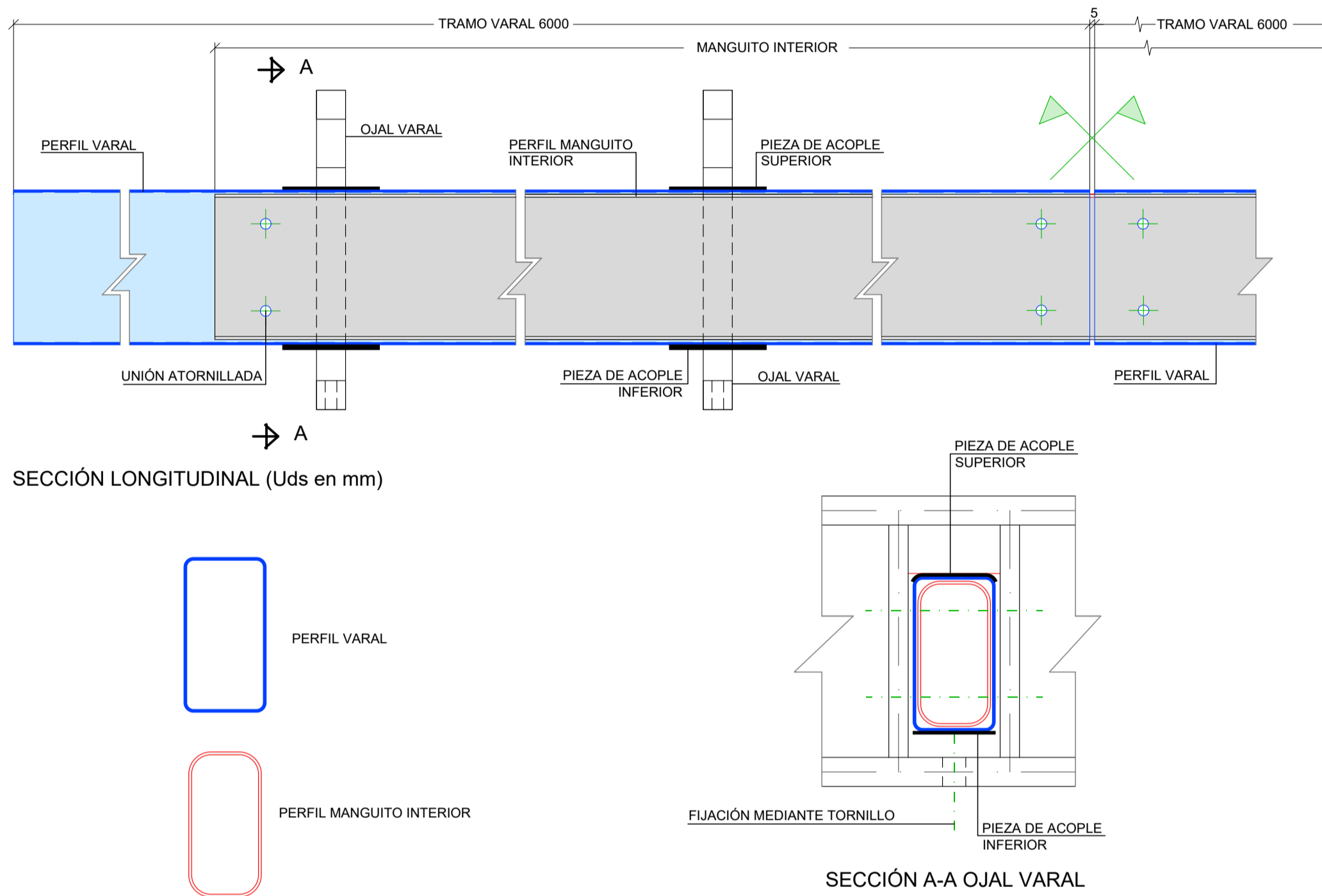
DETALLE MONTAJE DE VARALES MEDIANTE CONEXIÓN CON MANGUITO INTERIOR
