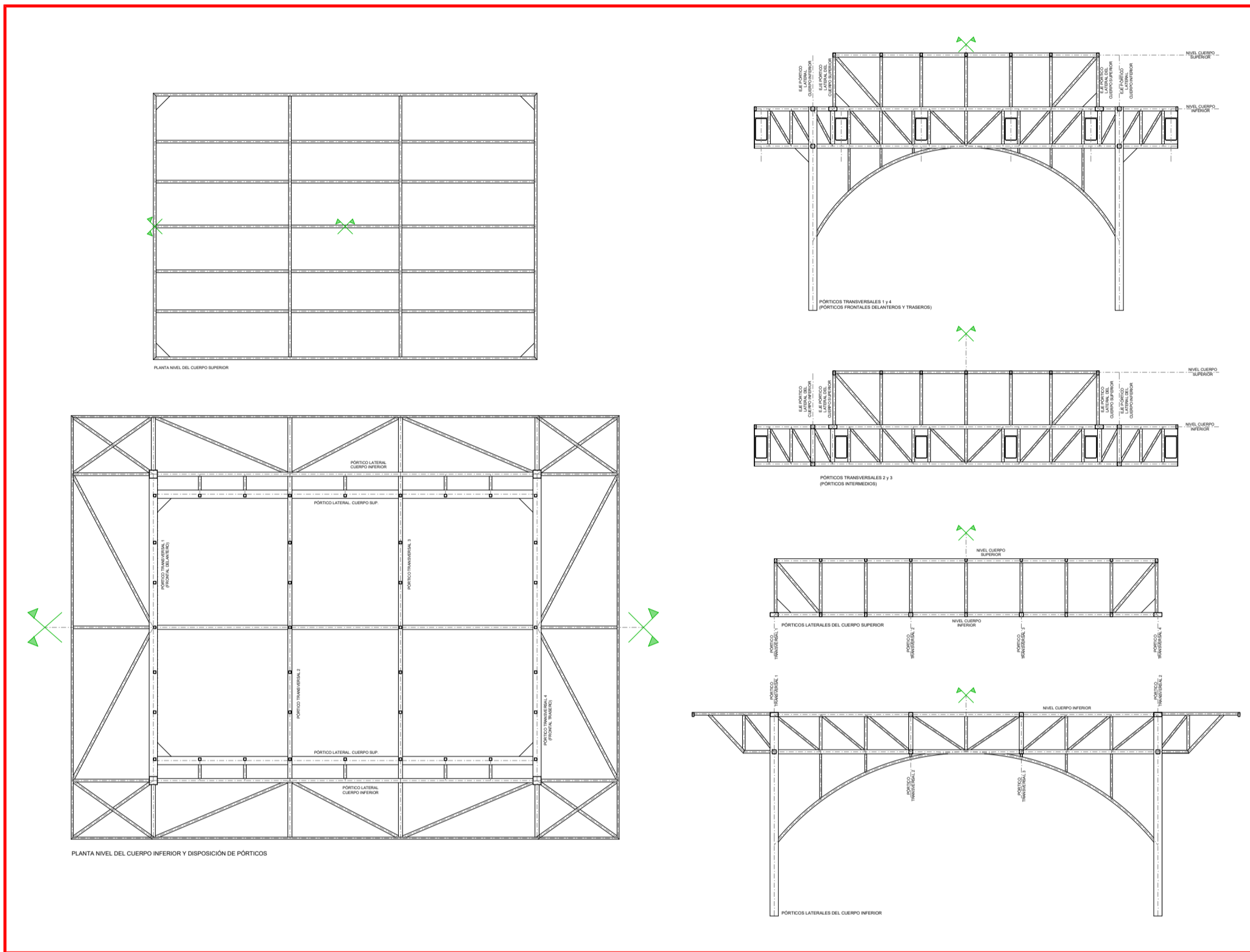
GEOMETRÍA DE PÓRTICOS Y NIVELES
